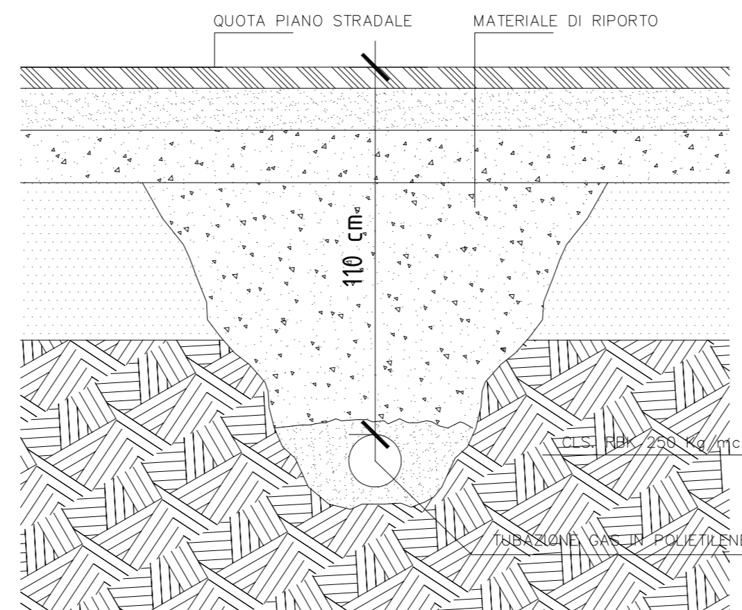
schema posa impianti scala 1:10
